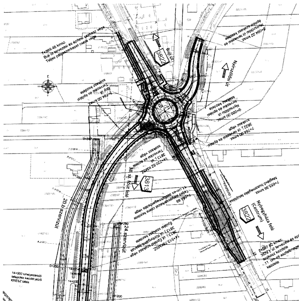
A Nyugati elkerülő út befejező csomópontjának tervezett átépítési helyszínrajza (részlet) Tervező: Cívis Komplex Mérnök Kft. (4030 Debrecen, Gizella u 13/D.)
