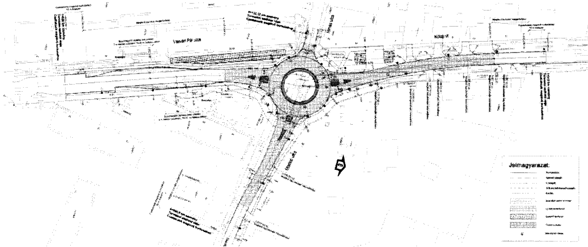
Vasvári Pál utca – Hímes utca – Kótaji út – Stadion utca közlekedési csomópont átépítési helyszínrajza Tervező: RODEN Mérnök Iroda Kft. (1089 Budapest VIII, Villám u. 13.)
