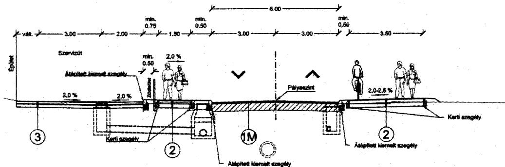
Vasvári Pál utca – Hímes utca – Kótaji út – Stadion utca közlekedési csomópont mintakeresztmetszelvényei Tervező: RODEN Mérnök Iroda Kft. (1089 Budapest VIII, Villám u. 13.)
