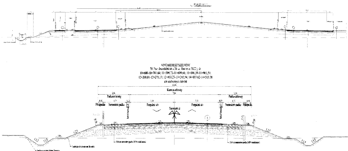
A Nyugati elkerülő út befejező csomópontjának tervezett mintakeresztszelvényei Tervező: Cívis Komplex Mérnök Kft. (4030 Debrecen, Gizella u 13/D.)
