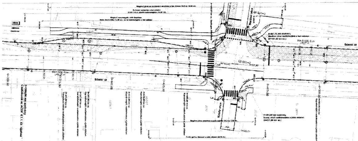
Stadion utca – Sóstói út - Krúdy Gyula utca közlekedési csomópont átépítési helyszínrajza Tervező: RODEN Mérnök Iroda Kft. (1089 Budapest VIII, Villám u. 13.)
