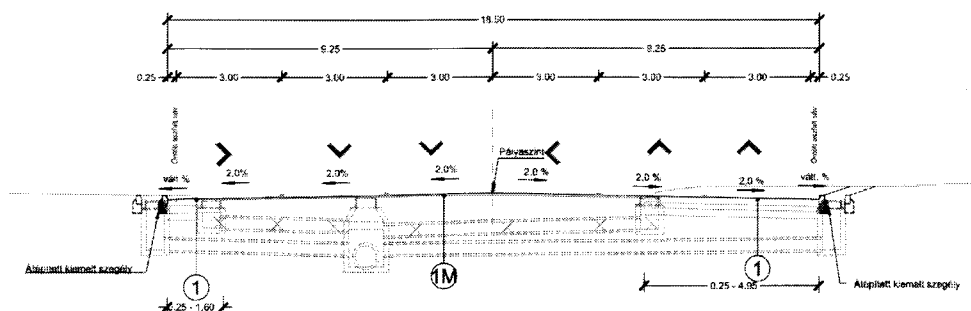
Stadion utca – Sóstói út - Krúdy Gyula utca közlekedési csomópont mintakeresztmetszései Tervező: RODEN Mérnök Iroda Kft. (1089 Budapest VIII, Villám u. 13.)
