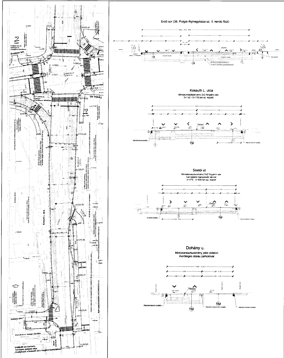
Sóstói út – Ferenc körút- Kossuth Lajos utca – Erdő sor és a Kossuth Lajos utca – Dohány utca közlekedési csomópontok átépítési helyszínrajza Tervező: RODEN Mérnök Iroda Kft. (1089 Budapest VIII, Villám u. 13.)
