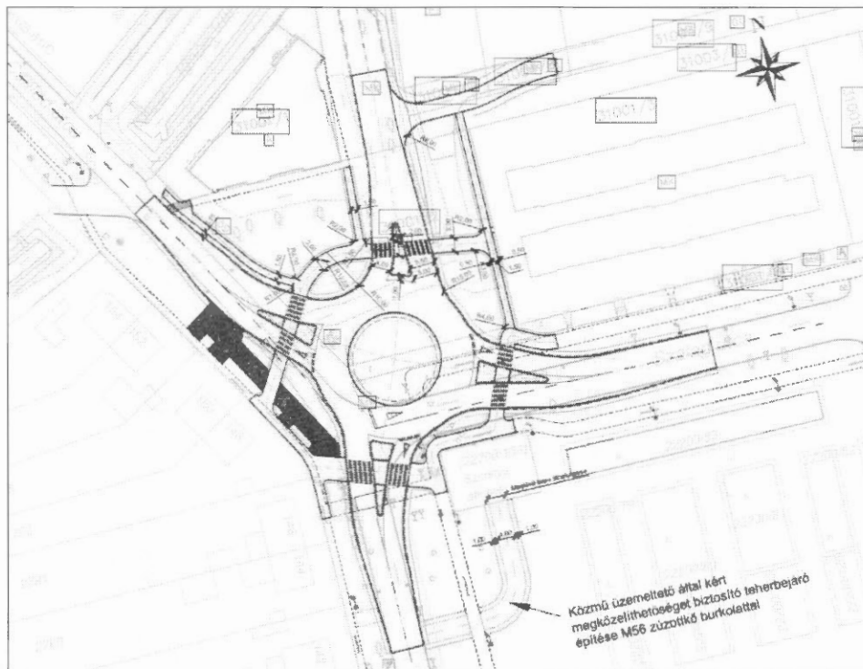
Család utca – Szalag utca csomópontja - Munkaközi forgalomtechnikai helyszínrajz Tervező: Cívis Komplex Mérnök Kft. (4030 Debrecen, Gizella u 13/D.)
