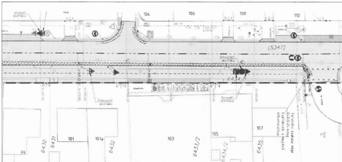
Szarvas utca, tervezett kerékpárút - Forgalmotechnikai helyszínrajz részlete Tervező: KÖZMŰTERV-M '93 Kft. (4400 Nyíregyháza, Selyem u. 21. B./1.)
