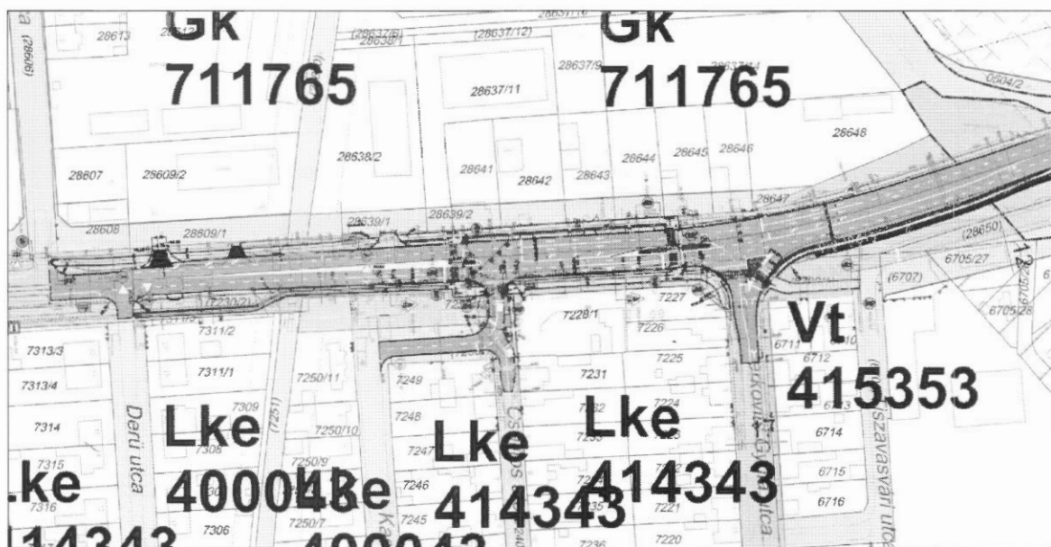
Tervezett csomópont szabályozási tervre illesztve
