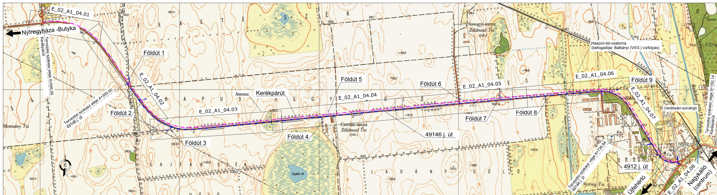
Nyíregyháza Déli ipari park fejlesztése – Átnézeti helyszínrajz Tervező: CÍVIS KOMPLEX MÉRNÖK Kft. (4034 Debrecen, Nagybánya u. 17.)
