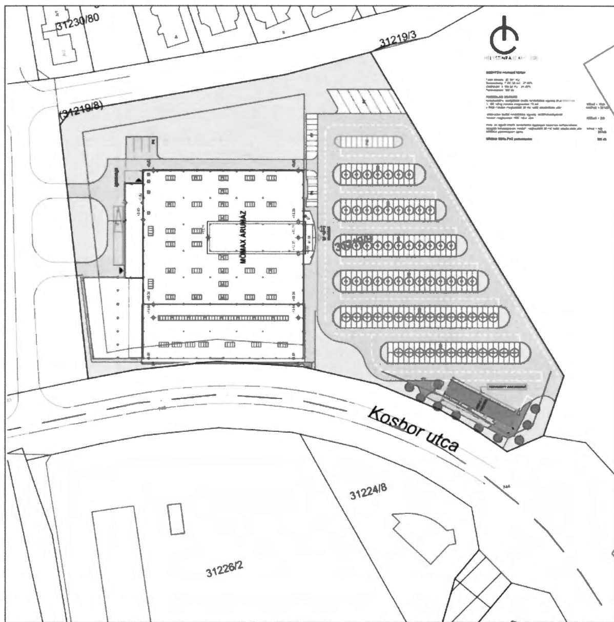
Nyíregyháza, Kosbor u. (hrsz.: 31219/9) tervezett helyszínrajz Tervező: Csikai Tibor, É 15-0409 – Archis 21 építésziroda Kft. (4431 Nyíregyháza, Pázsit u.12.)
