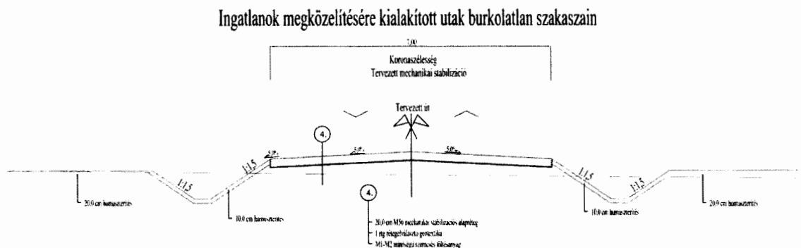
A Nyugati elkerülő út szervizútjainak tervezett mintakeresztmetszévei Tervező: Cívus Komplex Mérnök Kft. (4030 Debrecen, Gizella u 13/D.)
