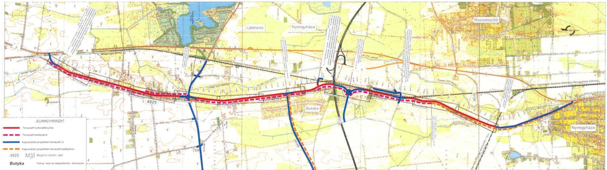
Nyíregyháza Déli ipari park fejlesztése – Átnézeti helyszínrajz Tervező: CIVIS KOMPLEX MÉRNÖK Kft. (4034 Debrecen, Nagybánya u. 17.)
