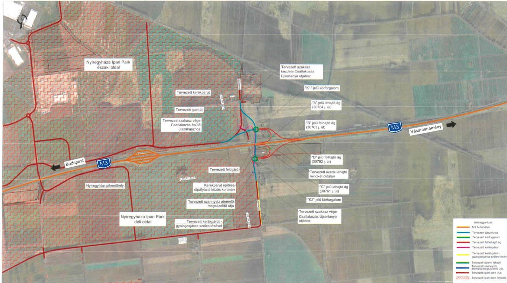
Nyíregyháza Ipari Park bővítése – M3 autópálya új külön szintű csomópont Tervező: CÍVIS KOMPLEX MÉRNÖK Kft. (4034 Debrecen, Nagybánya u. 17.)
