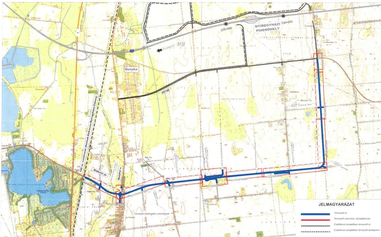
Nyíregyháza Megyei Jogú Város ipari park tervezési szolgáltatások – Déli ipari park fejlesztése – Átnézési helyszínrajz Tervező: CÍVIS KOMPLEX MÉRNÖK Kft. (4034 Debrecen, Nagybánya u. 17.)
